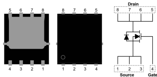
PDFN5x6
